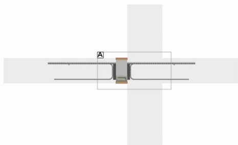
Roźmieszczenie elementów ogniochronnych
